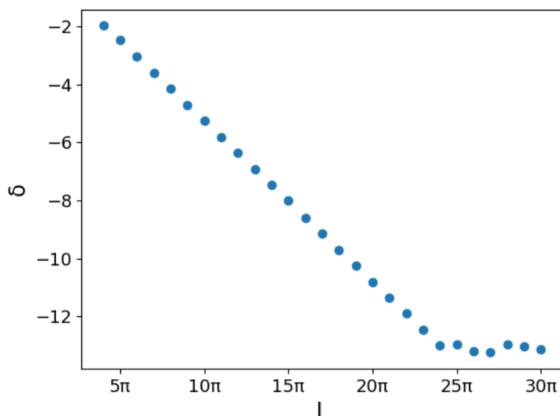
Рис. 1. Зависимость порядка ширины зоны СЗ системы Захарова – Шабата \delta от размера периодического ящика L .
