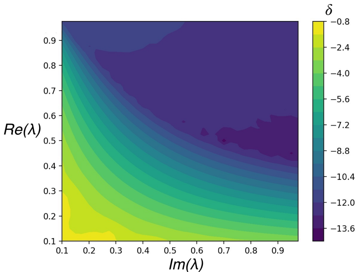
Рис. 2. Зависимость порядка ширины зоны СЗ системы Захарова – Шабата \delta от ее положения на комплексной плоскости.
